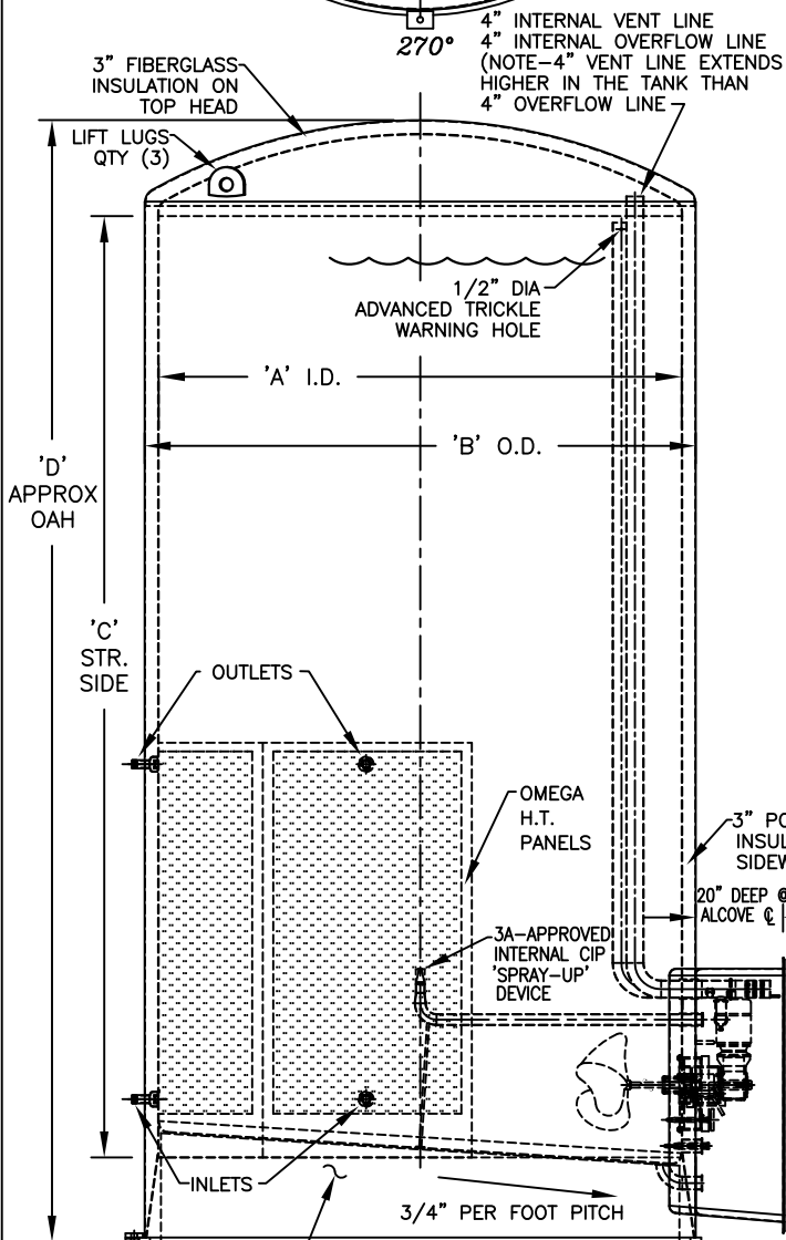
ELEVATION
